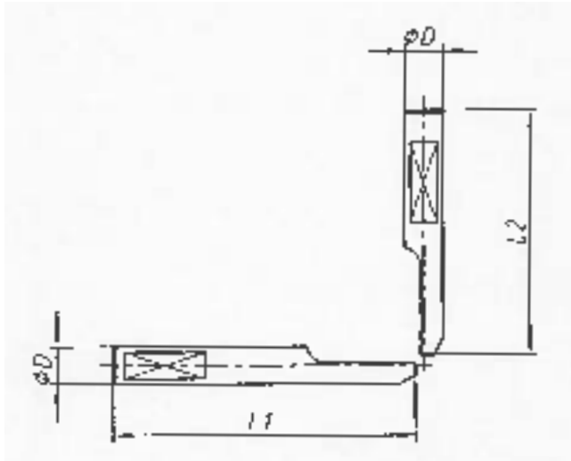
Bec du levier cliquet Nocken des Klink-Hebels Toe of ratchet lever
